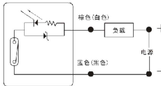
接线图
